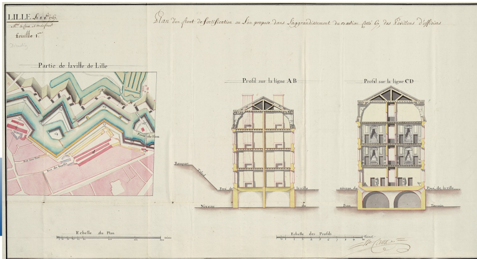
Place de Lille - bastion 67, pavillons d'officiers, 8/10/1767, 66 J 1356, Archives Départementales du Nord
