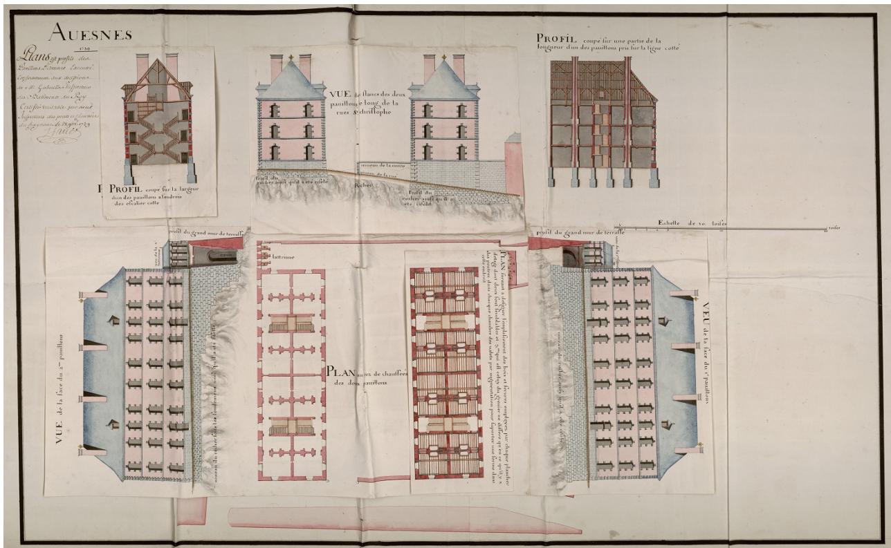
Place d'Avesnes-sur-Helpe - pavillons des officiers, 28/11/1739, C 10594, Archives Départementales du Nord
